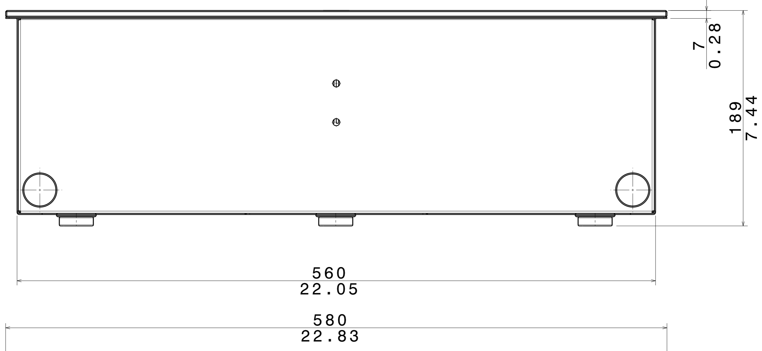
Vista dal basso Scala: 1:2
