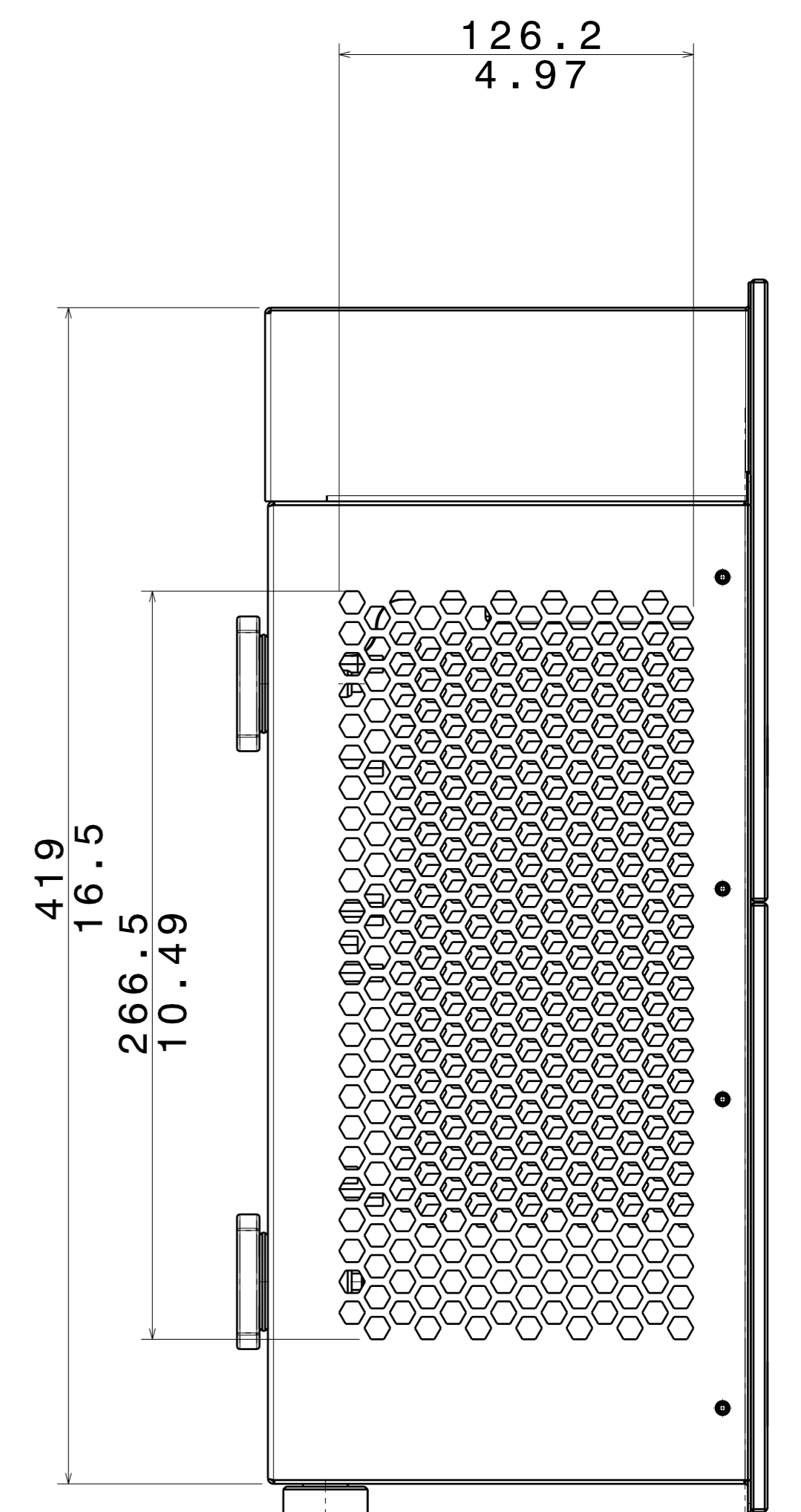
Vista da sinistra Scala: 1:2
