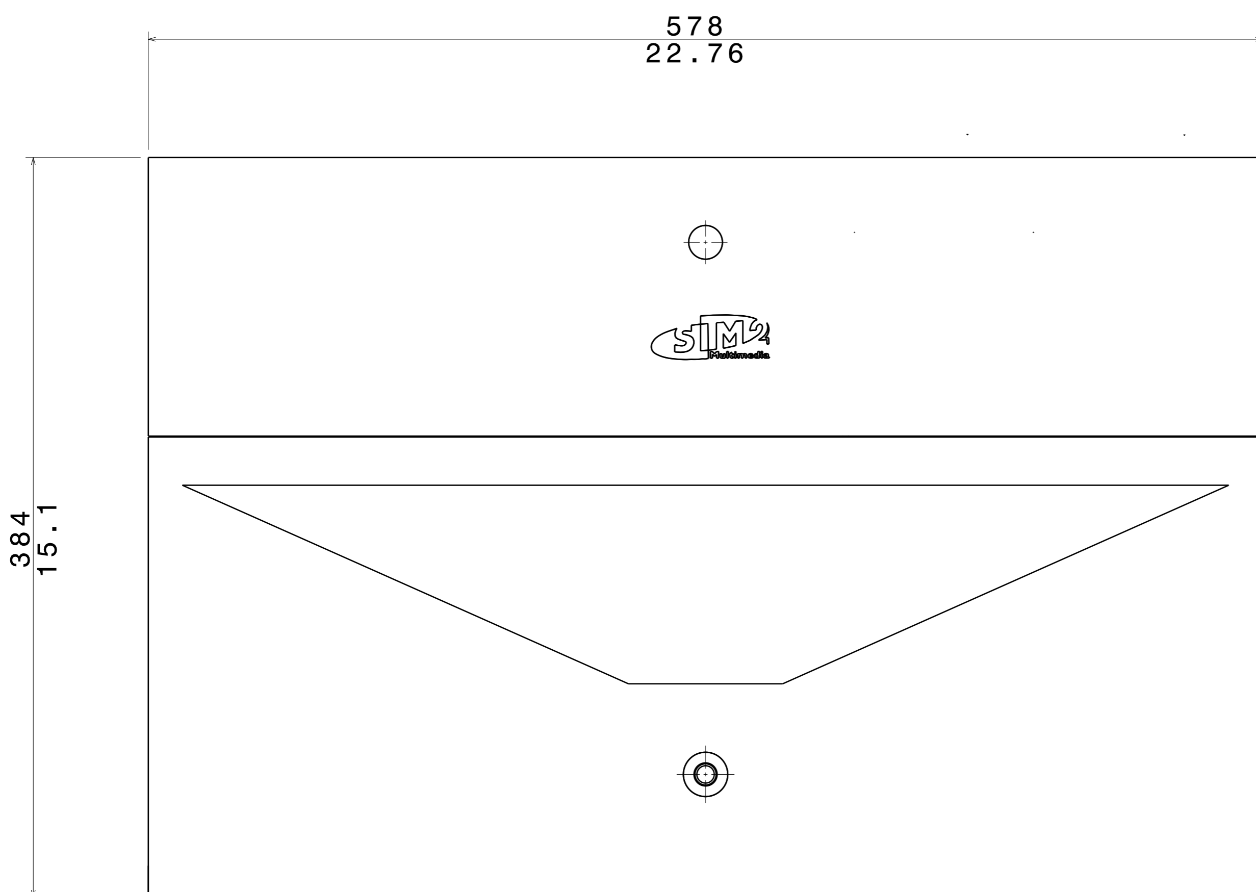
Vista posteriore Scala: 1:2
