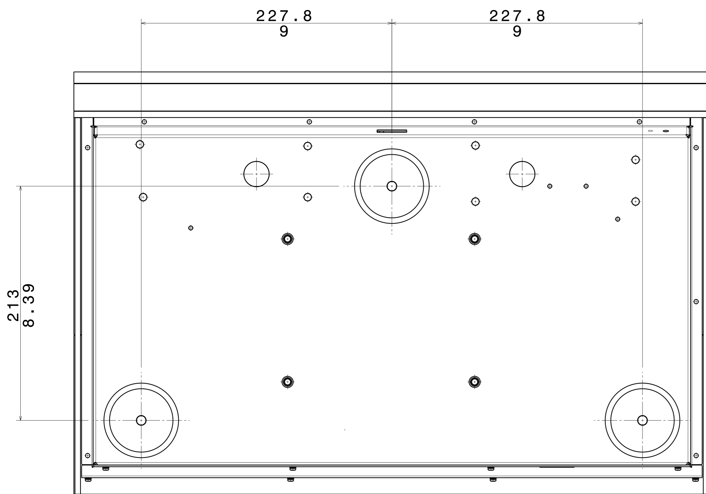
Vista frontale Scala: 1:2
